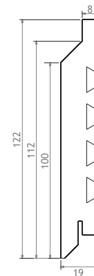
perfil Channel*
