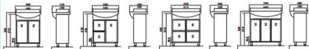
Мобис 50 / Mobis 50 Тумба с умывальником Cabinet with washbasin
