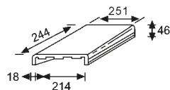
Pasamanos int. 21,5 Handrail int. 21,5 Cod. 00007
