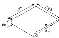
Remate natural de 33 Natural edge Cod. 00197
