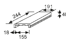
Pasamanos int. 15,5 Handrail int. 15,5 Cod. 00016
