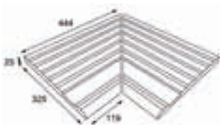
Esq. int. remate desbordante Overflowing internal edge Cod. 01931
