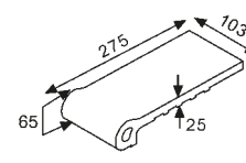
Remate natural de 10 Natural edge Cod. 00194
