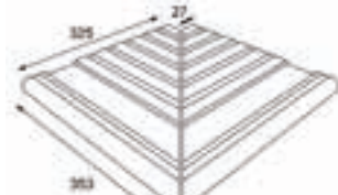
Esq. ext. remate desbordante Overflowing external edge Cod. 01932
