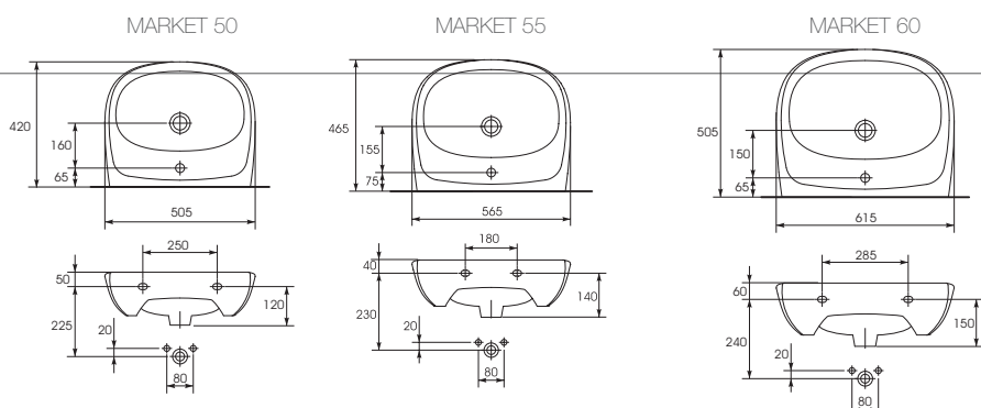
Раковина MARKET 50, 55. С отверстием или без отверстия для арматуры, монтаж с пьедесталом. Размер: 50x42 см / 56x46 см
