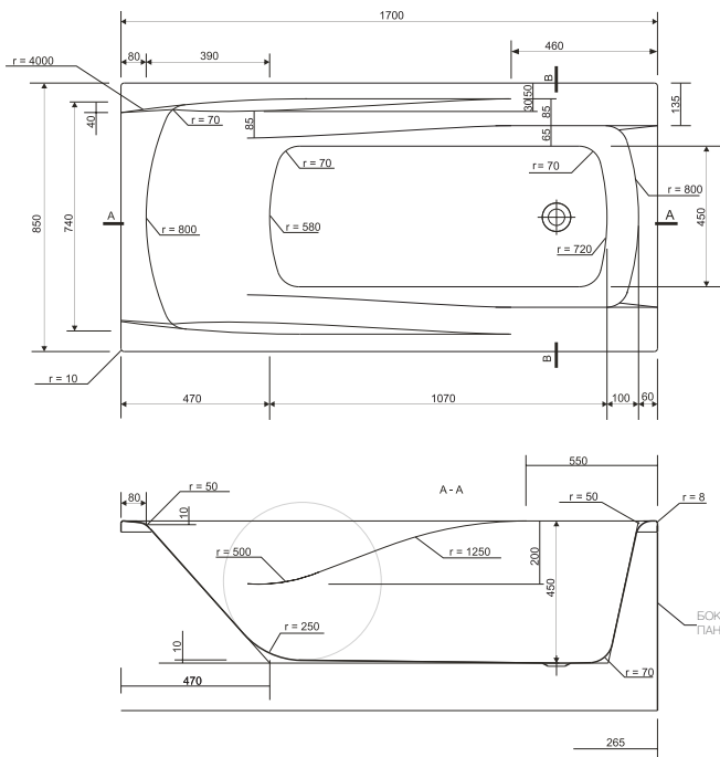
ZEN 170
