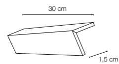
PERFIL 1,5x30 RECT [ 1,5x29,5x0,90 cm ] P20 /peça_piece
