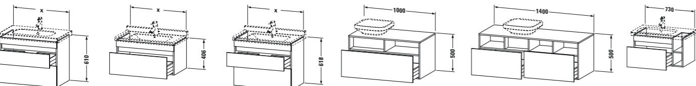
# DS 6483 ↔ 600 mm # DS 6387 ↔ 650 mm # DS 6487 ↔ 650 mm # DS 6784 L/R ↔ 1000 mm # DS 6785 L/B/R ↔ 1400 mm # DS 6394 → D-Code # 034265 → Starck 3 # 030470 → Starck 3 # 030470 → ↗ 550 mm → ↗ 550 mm → DuraStyle # 232580 # DS 6484 ↔ 800 mm # DS 6388 ↔ 800 mm # DS 6488 ↔ 800 mm # DS 6388 ↔ 800 mm # DS 6488 ↔ 800 mm # DS 6388 ↔ 800 mm → D-Code # 034285 → Starck 3 # 030480 → Starck 3 # 030480 → Starck 3 # 030480 → Starck 3 # 030480 → Starck 3 # 030480 # DS 6485 ↔ 1000 mm # DS 6389 ↔ 1000 mm # DS 6489 ↔ 1000 mm # DS 6489 ↔ 1000 mm # DS 6489 ↔ 1000 mm # DS 6489 ↔ 1000 mm → D-Code # 034210 → Starck 3 # 030410 → Starck 3 # 030410 → Starck 3 # 030410 → Starck 3 # 030410 → Starck 3 # 030410 # DS 6486 ↔ 1200 mm # DS 6390 ↔ 1200 mm # DS 6490 ↔ 1200 mm # DS 6490 ↔ 1200 mm # DS 6490 ↔ 1200 mm # DS 6490 ↔ 1200 mm → D-Code # 034212 → Starck 3 # 030412 → Starck 3 # 030412 → Starck 3 # 030412 → Starck 3 # 030412 → Starck 3 # 030412 ↗ 448 mm ↗ 448 mm ↗ 448 mm ↗ 448 mm ↗ 448 mm ↗ 448 mm
