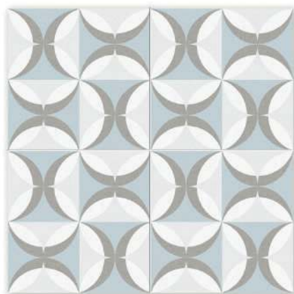
NARBONNE BLUE GT5 45 x 45 CM ( PRE-CUT 22,5 x 22,5 CM ) R10 FINISH (C2) PEI III · MOHS 8
