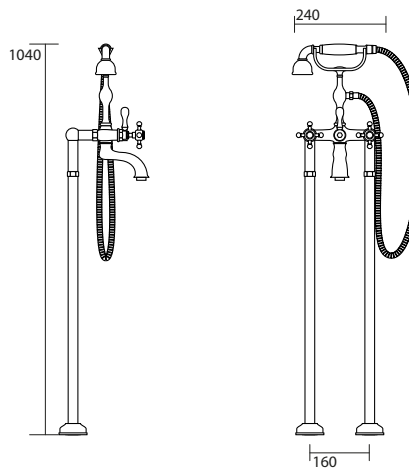
7395 Coppia colonnine cm 80 per attacco a pavimento Pair of columns cm 80 for floor assembling
