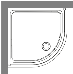
9151 Cabina doccia semicircolare DX/SX per piatto doccia semicircolare 90x90h.187 Corner reversible shower enclosure for corner shower-tray 90x90x187
