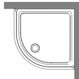
9158 Cabina doccia semicircolare DX/SX per piatto doccia semicircolare 80x80h.187 Corner reversible shower enclosure for corner shower-tray 80x80x187
