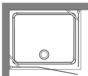
9141 Cabina doccia DX con porta battente in linea e fisso laterale per piatto doccia 80x96 DX apertura lato 96. Right shower enclosure with door for right shower-tray 80x96 opening on 96 side Usable opening 54 cm, height 180 cm.
