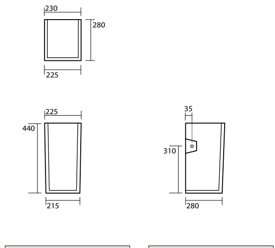
3575 Semi-colonna Semi-pedestal
