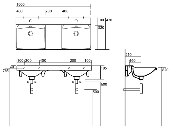
3404 "BUDDY" Lavabo doppia vasca 100x42 sospeso, appoggio monoforo "BUDDY" One hole wall hung or counter top double basin 100x42
