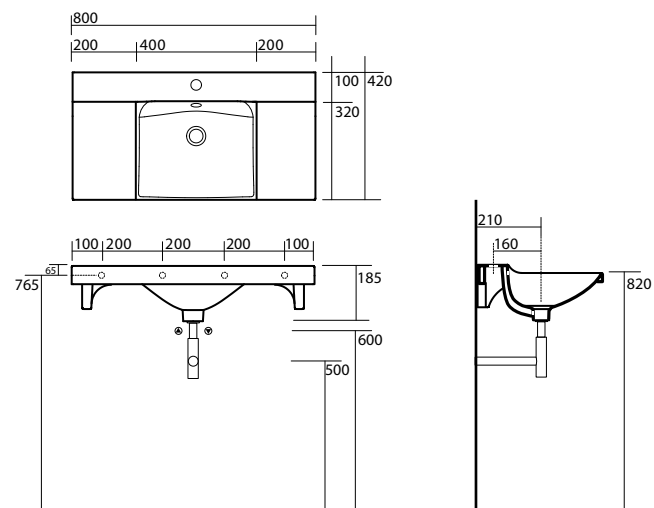
3403 "BUDDY" Lavabo 80x42 sospeso, appoggio monoforo "BUDDY" One hole wall hung or counter top washbasin 80x42
