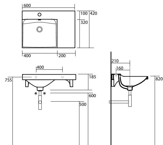
3402 "BUDDY" Lavabo 60x42 sospeso, appoggio monoforo "BUDDY" One hole wall hung or counter top washbasin 60x42
