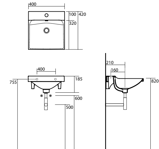
3401 "BUDDY" Lavabo 40x42 sospeso, appoggio monoforo "BUDDY" One hole wall hung or counter top washbasin 40x42
