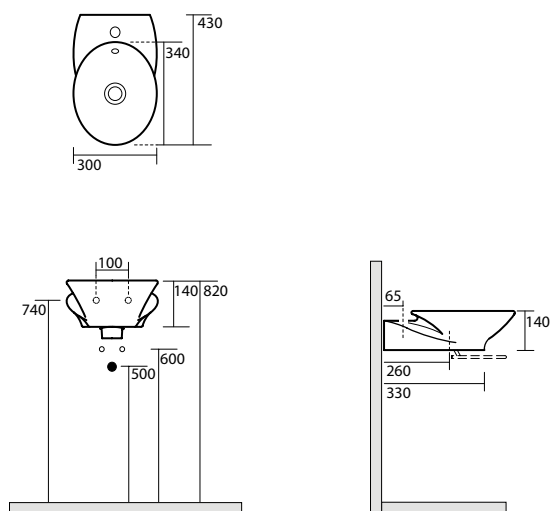
3420 "SWAN" lavabo 30x43 sospeso o appoggio monoforo "SWAN" one hole wall hung or counter top washbasin 30x43
