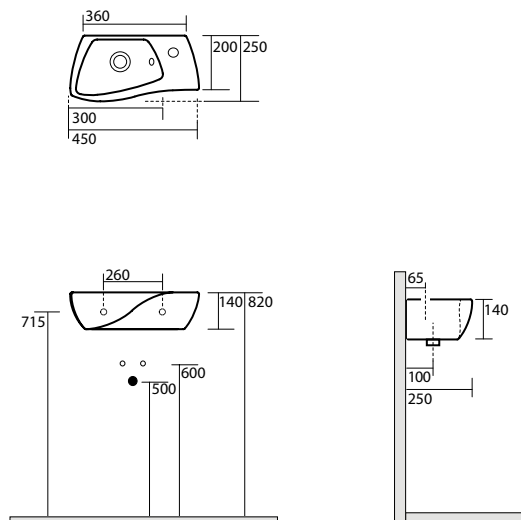
3421 "WAVE" lavabo 45x25 sospeso o appoggio monoforo "WAVE" one hole wall hung or counter top washbasin 45x25
