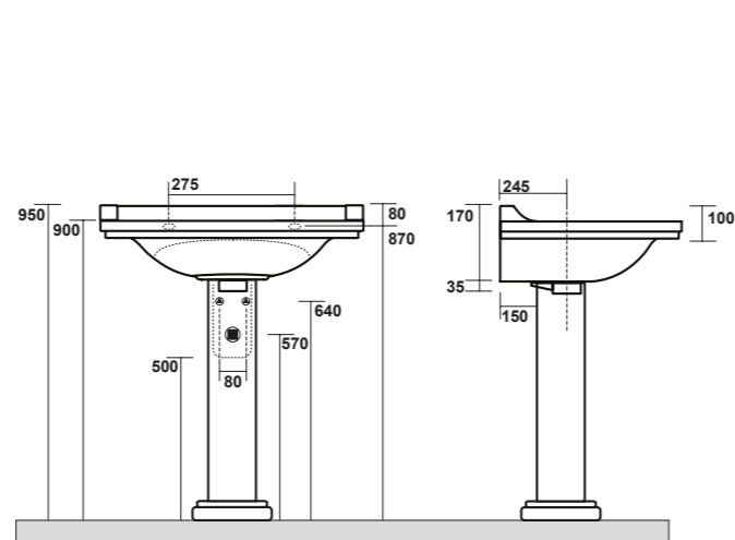
4170 Colonna Pedestal
