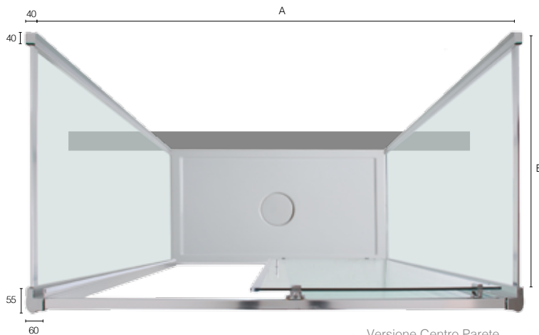
Versione Centro Parete Center Wall Version
