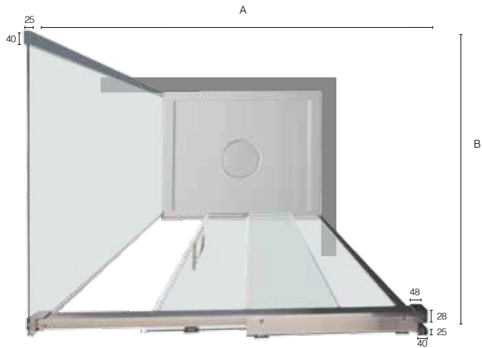
Versione Angolare DX da 900 mm Right Corner Version 900 mm
