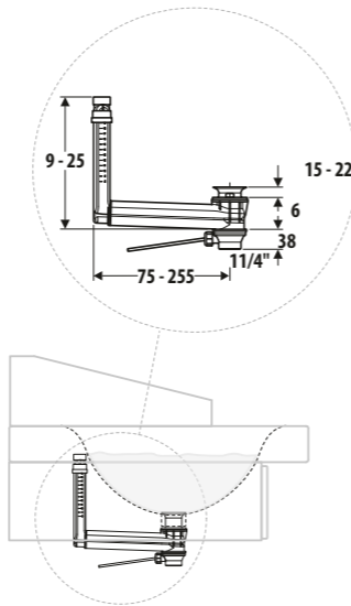
7530 Piletta con troppo pieno per lavabi Drive plug w/overflow for washbasin
