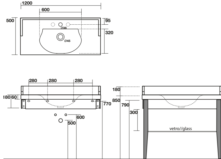
3935 Lavabo con alzata cm L.120xP.50 (3 fori a richiesta) Washbasin w/upstand cm L.120xP.50 (3 holes on demand )
