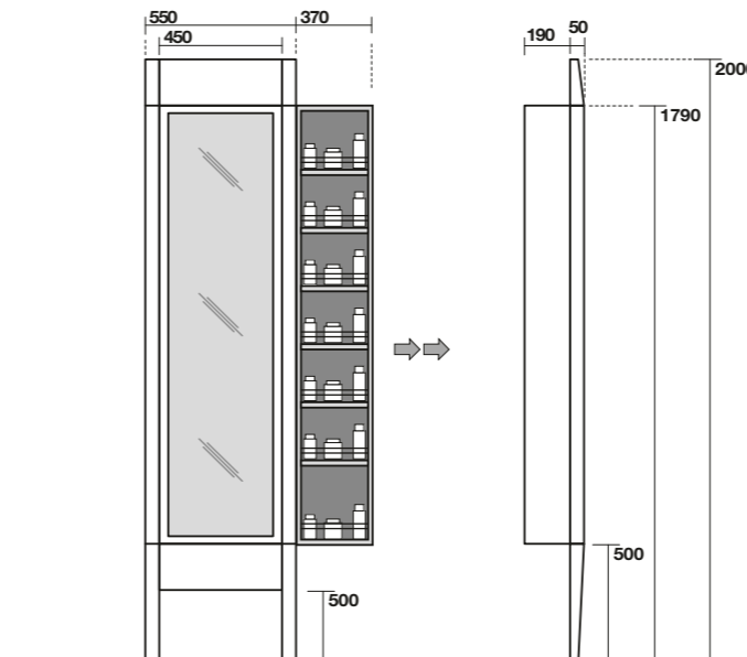
9183 Specchio a terra con contenitore estraibile cm L.55xH.200xP.24 Mirror cabinet w/hideaway shelves cm L.55xH.200xP.24
