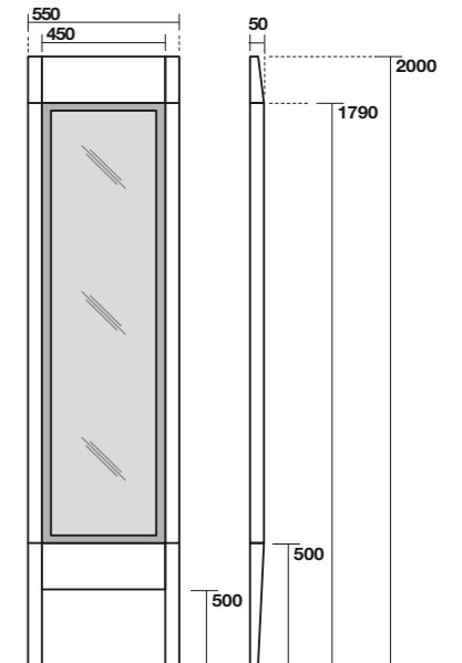
9182 Specchio a terra cm L.55xH.200 Floor standing mirror cm L.55xH.200
