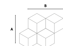
A 30,5 cm - 12" B 35,2 cm - 13 7/8"
