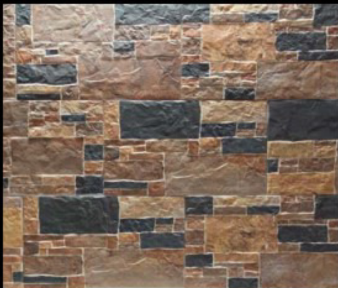
Pluton Caldera
