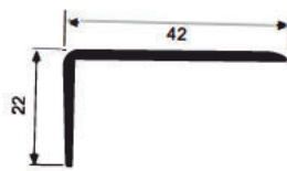
42x22 ЛЕСТНИЦА
