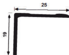
25X19 ЛЕСТНИЦА
