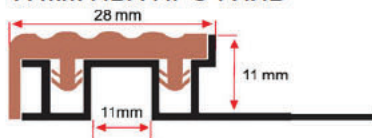
11 mm ПВХ ПРОФИЛЬ
