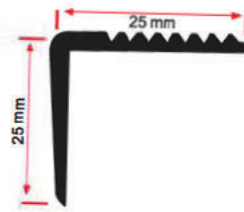
25X25 ЛЕСТНИЦА
