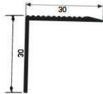
30X30 ЛЕСТНИЦА
