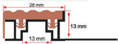
13 mm ПВХ ПРОФИЛЬ
