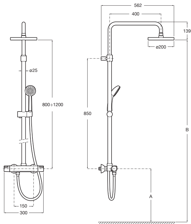
Instalación regulable de 800 a 1200 mm Adjustable installation from 800 to 1200 mm Installation réglable de 800 à 1200 mm Регулируемая высота от 800 до 1200 мм.
