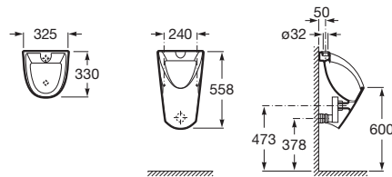
Urinoir à alimentation supérieure. Писсуар с верхним подводом.
