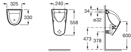
Urinoir à alimentation postérieure. Писсуар с задним подводом.
