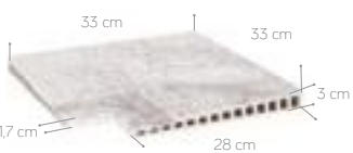
ÁNGULO DESBORDANTE C-3 33 x 33 cm - 13.0' x 13.0'
