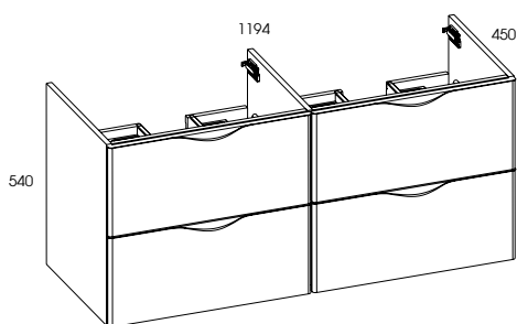
szafka podumywalkowa 120 4S • unit 120 4DR
