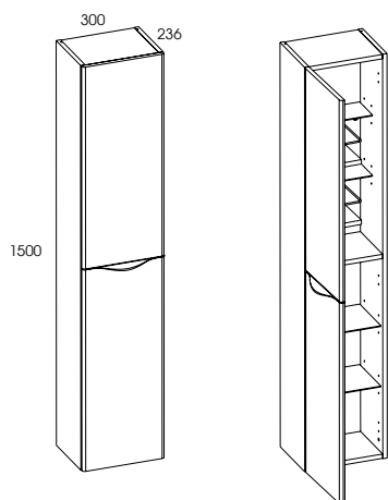
ślupek 30 1D LEWY • column 30 1D LEFT
