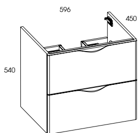
szafka podumywalkowa 60 2S • unit 60 2DR
