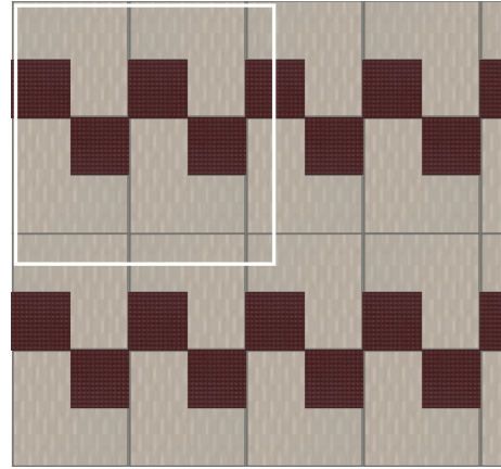
PIECES 1 m 2 6_D.SOLAIRE TAUPE LINE-2/44,9 5_D.SOLAIRE BORDEAUX SQUARE-4/22,3 (joint 2 mm)
