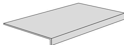
Lineare ad Elle - L-shaped element 30,2x60,4x5 - 12"x24"x2 Naturale/Rettificato - Matte/Rectified
