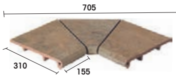
CARTABÓN INTERIOR BORDE PISCINA RECTO (*)
