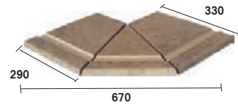
CARTABÓN EXTERIOR BORDE PISCINA TÉCNICO (*)
