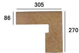
ZANQUÍN RECTO PLUS
