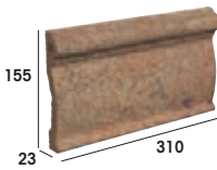
REMATE DE FRISO
